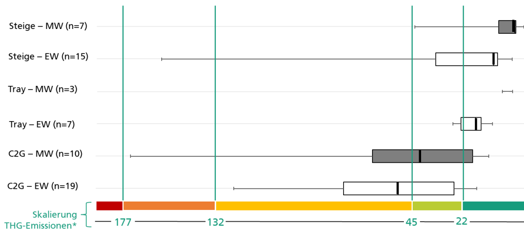
Abbildung 2: Ergebnisse einer Metaanalyse zu den Treibhausgasemissionen von Mehrweg- und Einwegsystemen (* In kg CO 2 -Äq pro Umlauf und 1000 L verpacktes Volumen. Das Volumen der Pflanzentrays bezieht sich auf das errechnete Volumen aller Pflanzentöpfe, die in das jeweilige Tray passen. Die Daten wurden als Boxplot dargestellt. Dabei ist der Wert ganz links der Maximalwert, der ganz rechts der Minimalwert. Der senkrechte Strich in der Mitte stellt den Median dar und die Box um den Median umfasst die 25 Prozent der Daten, die oberhalb und unterhalb des Medians liegen. Eine detaillierte Erklärung zum Boxplot findet sich hier: https://en.wikipedia.org/wiki/Box_plot )
